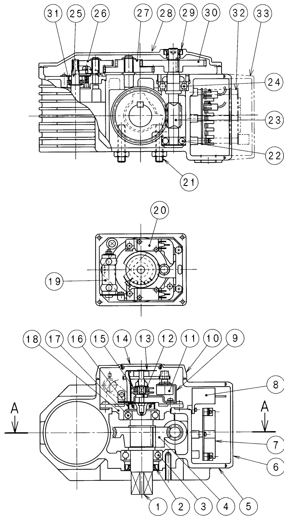
断面 A-A
